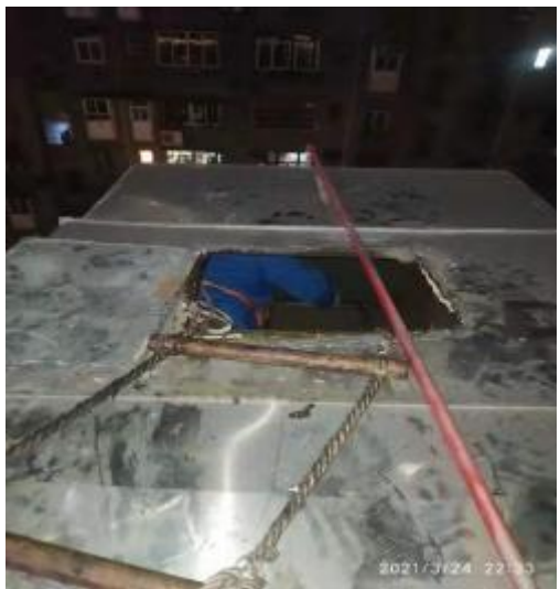
6楼平台竖管施工中
