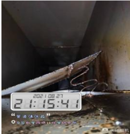
管道清洗前
