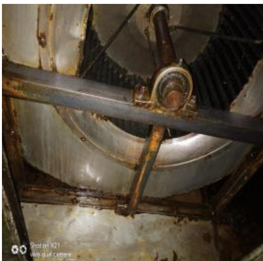
3楼平台风机清洗后 3
