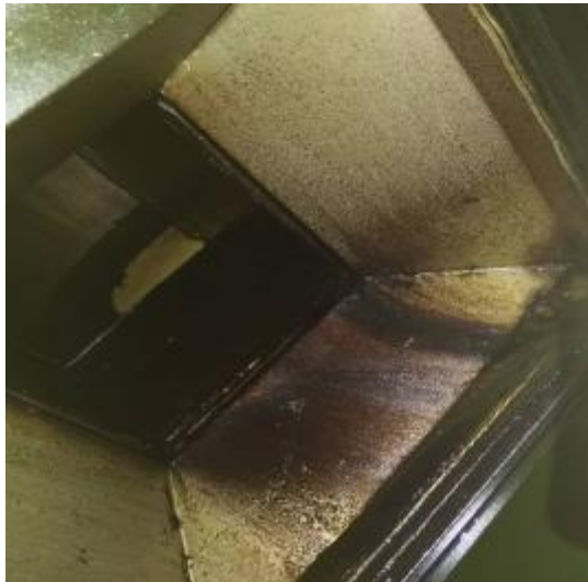
主管道清洗前
