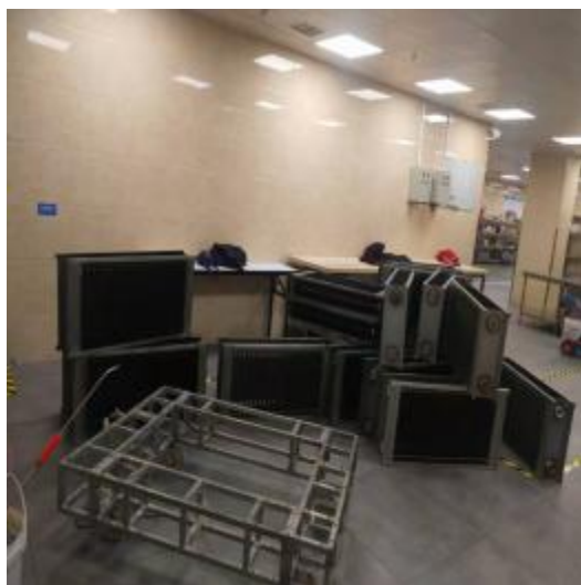
中厨房，员工厨房，烧烤房净化器清洗前
